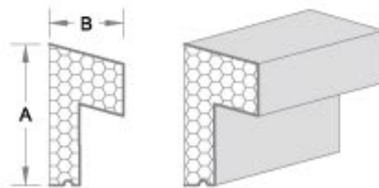
产品编号,CK024 A: 12.07cm B: 6.35cm
