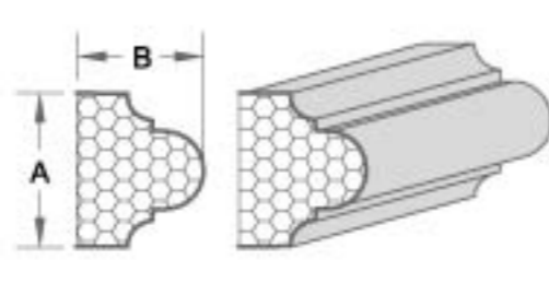
产品编号:XB030 A: 7.62cm B: 6.35cm
