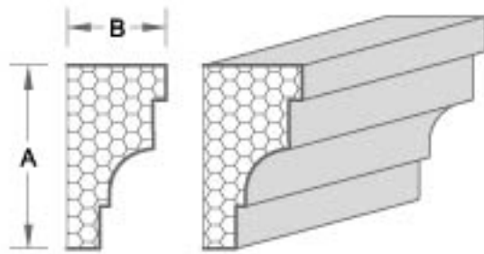
产品编号:XB016 A: 10.48cm B: 5.08cm
