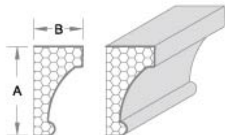
产品编号: YK056 A: 33.02cm B: 17.78cm
