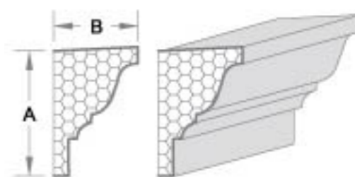
产品编号:YK012 A: 19.69cm B: 12.7cm
