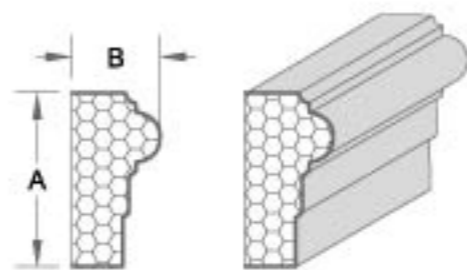
产品编号:XB037 A: 16.35cm B: 8.26cm
