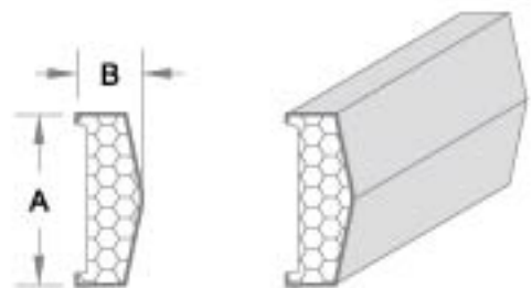
产品编号:QM002 A: 40.64cm B: 15.88cm
