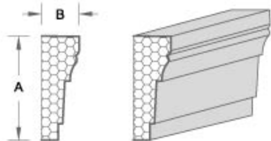
产品编号:XB009 A: 13.97cm B: 5.08cm
