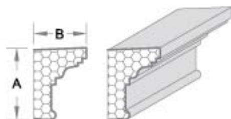
产品编号: YK051 A: 20.96cm B: 15.24cm
