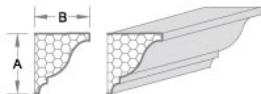
产品编号:YK019 A: 13.34cm B: 12.07cm
