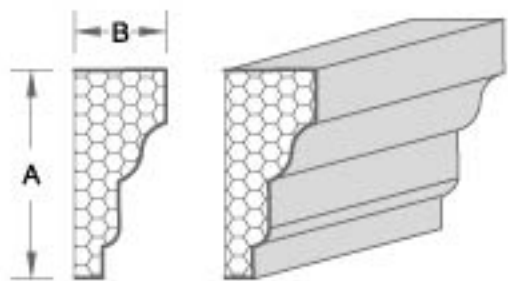
产品编号:XB014 A: 16.19cm B: 6.99cm
