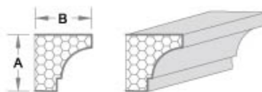
产品编号:YK013 A: 8.26cm B: 8.26cm
