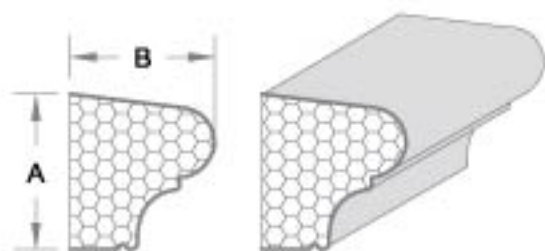
产品编号,CK026 A: 16.51cm B: 15.24cm
