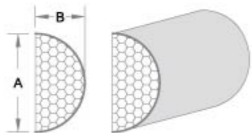
产品编号: LZ032 A: 38.10cm B: 19.05cm
