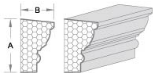
产品编号:YK017 A: 19.69cm B: 12.38cm
