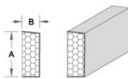
产品编号:XB069 A: 30.48cm B: 11.43cm
