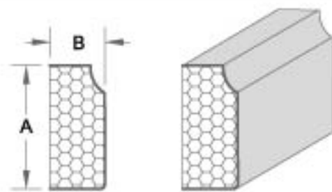
产品编号: MJ008 A: 11.43cm B: 5.08cm
