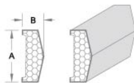
产品编号:QM013 A: 38.10cm B: 15.68cm
