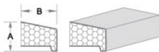
产品编号,CK015 A: 15.24cm B: 16.42cm
