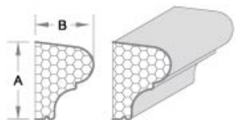
产品编号,CK027 A: 16.19cm B: 12.07cm
