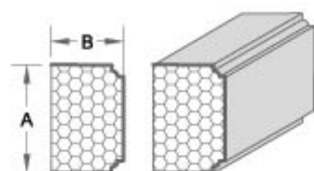
产品编号:XB044 A: 22.86cm B: 15.24cm
