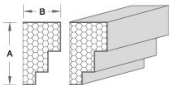
产品编号:XB012 A: 9.53cm B: 5.72cm
