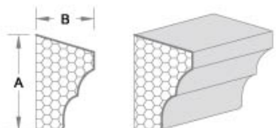
产品编号,CK022 A: 10.80cm B: 6.67cm
