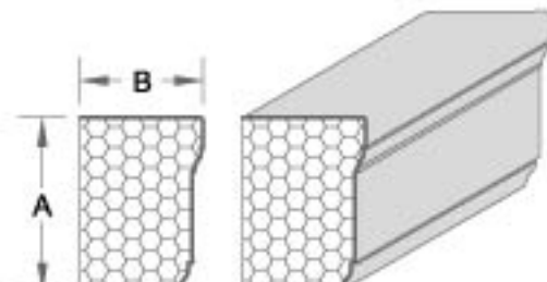
产品编号:XB052 A: 15.24cm B: 10.80cm
