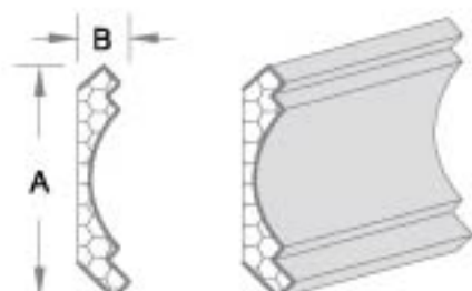
产品编号:YK022 A: 26.04cm B: 5.72cm
