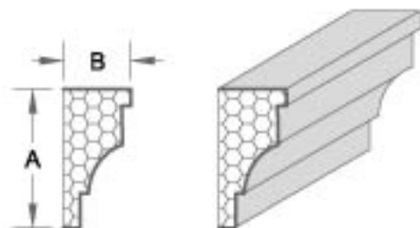
产品编号:XB061 A: 15.24cm B: 7.46cm
