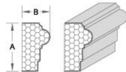
产品编号:XB040 A: 14.45cm B: 8.26cm
