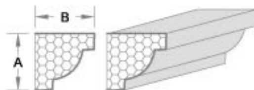
产品编号:YK003 A: 9.20cm B: 9.53cm
