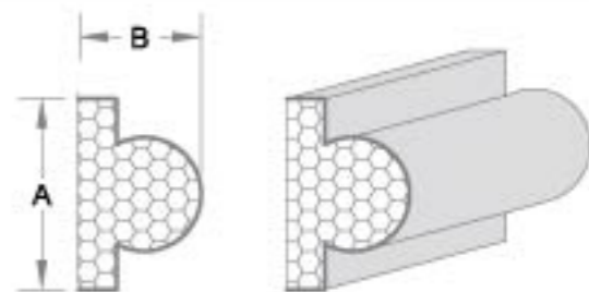
产品编号: LZ037 A: 38.10cm B: 12.38cm
