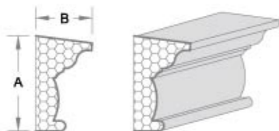
产品编号:CY002 A: 12.07cm B: 7.14cm
