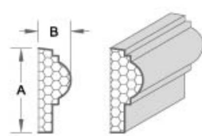
产品编号:XB034 A: 26.67cm B: 10.16cm
