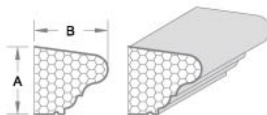
产品编号,CK028 A: 15.24cm B: 16.51cm
